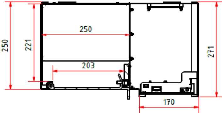
D-D ( 1 : 5 )
